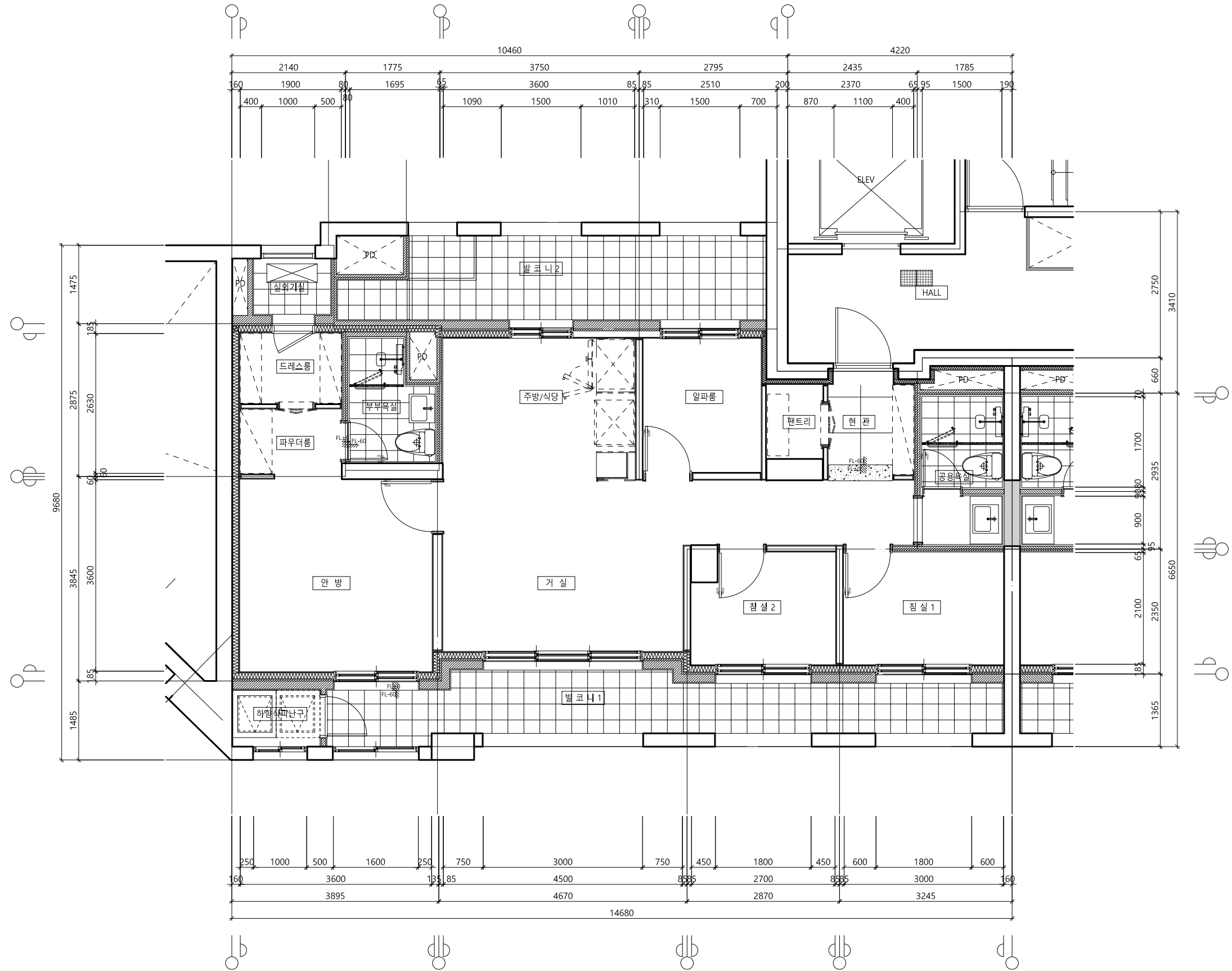
1 A 84m² 단위세대평면도(기본형) SCALE : A1= 1 / 40 A3= 1 / 80
