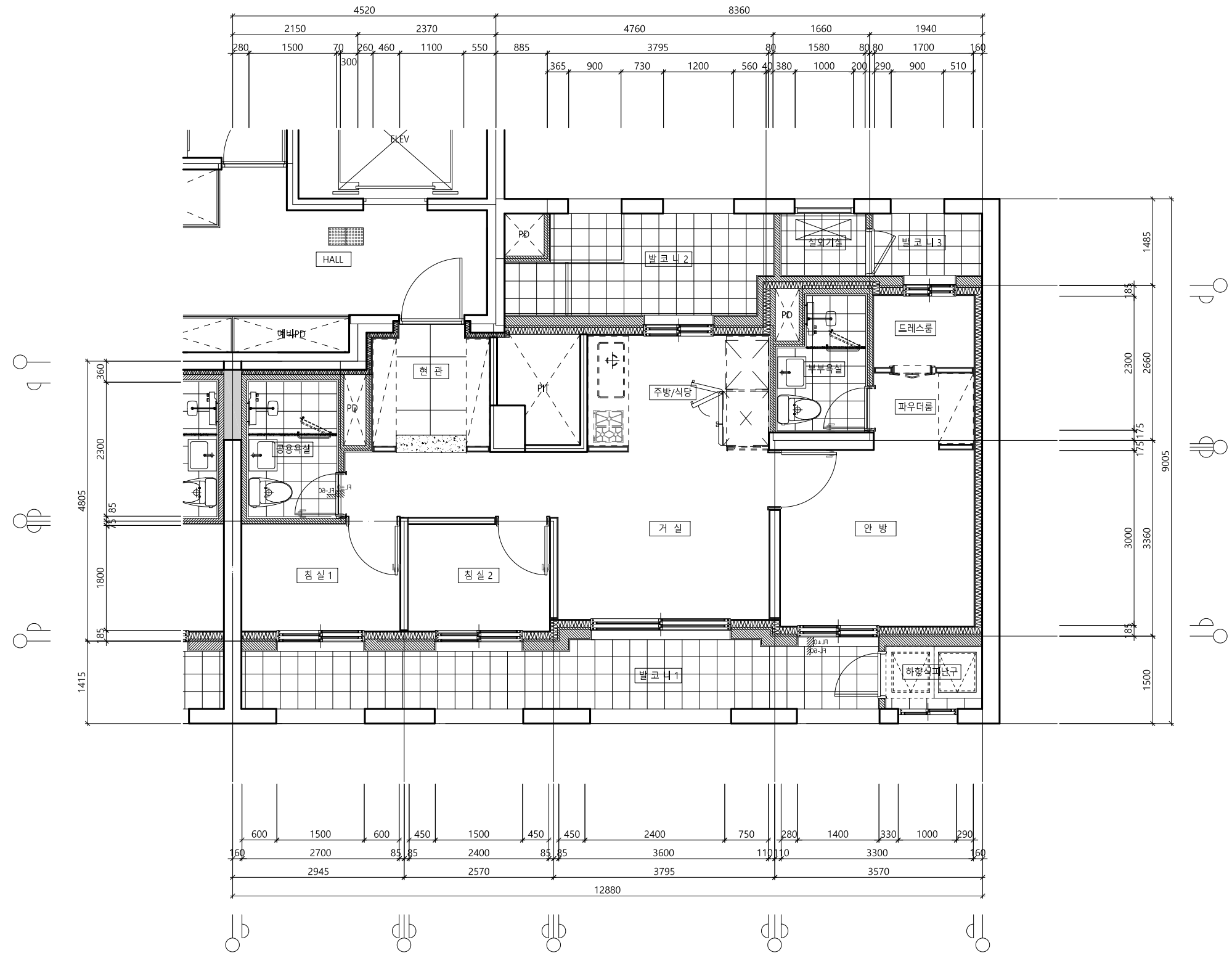
59Am 2 단위세대평면도(기본형) SCALE : A1= 1 / 40 A3= 1 / 80
