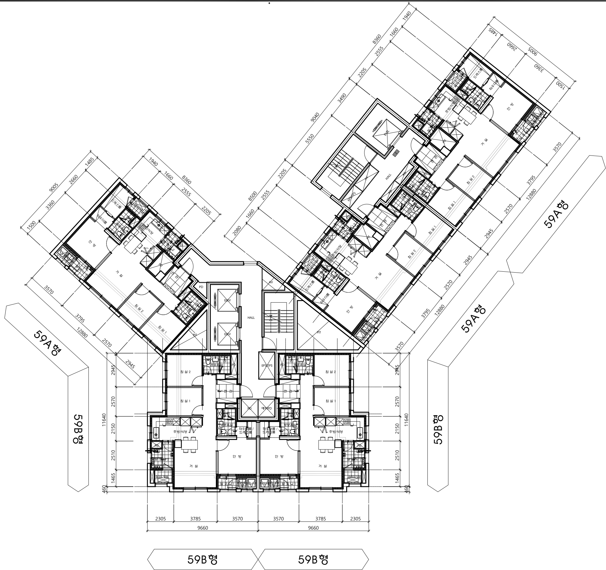
102동 기준층 평면도 SCALE : A1= 1 /100 A3= 1 /200
