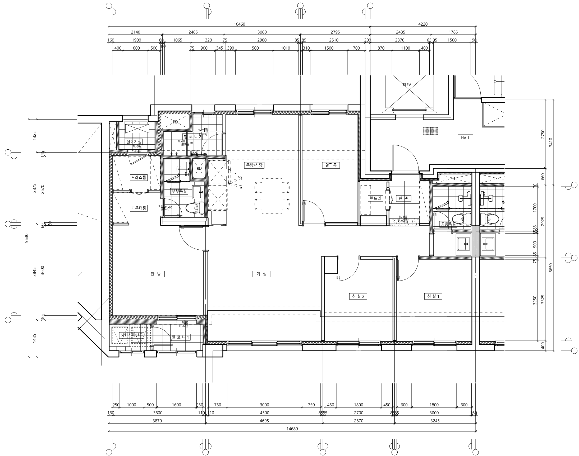
1 A 84m² 단위세대평면도(확장형) SCALE : A1= 1 / 40 A3= 1 / 80
