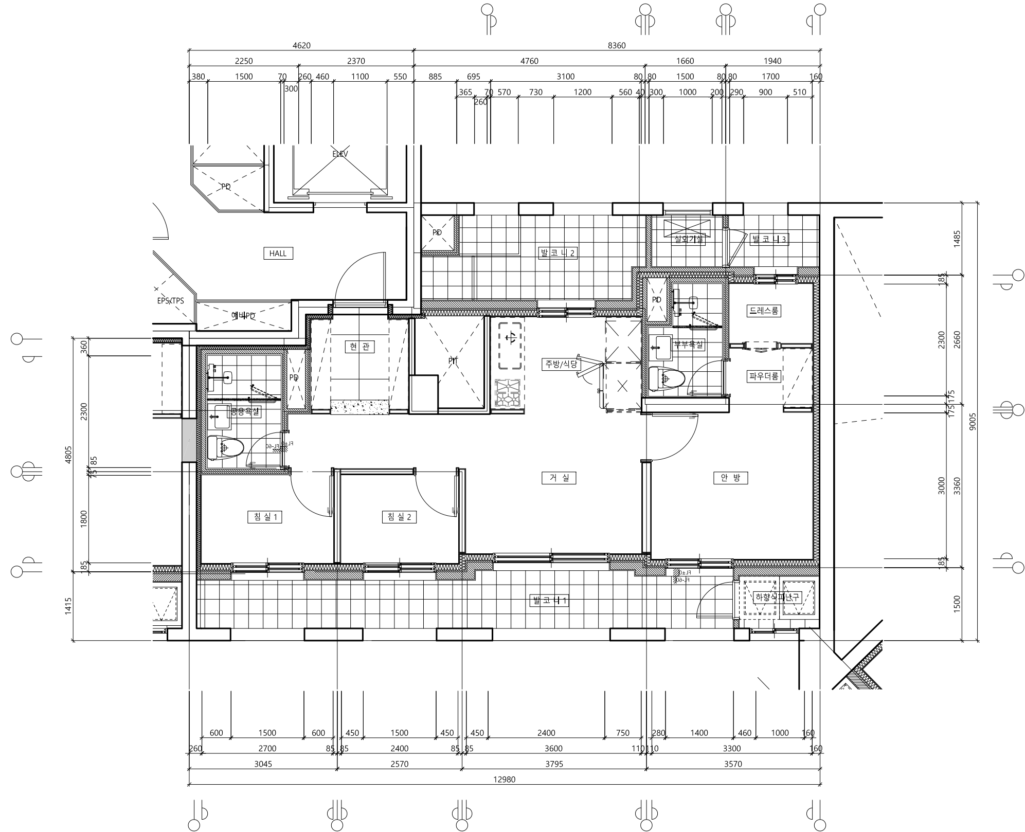
1 A 59Cm 2 단위세대평면도(기본형) SCALE : A1= 1 / 40 A3= 1 / 80
