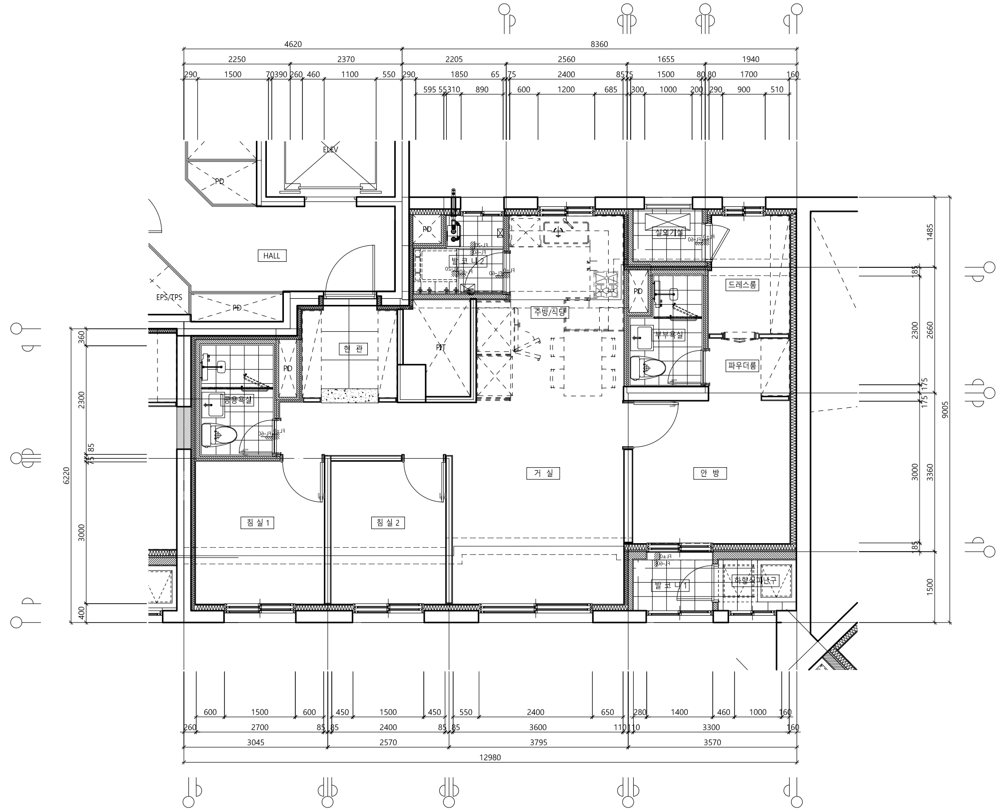
59Cm² 단위세대평면도(확장형) SCALE : A1= 1 / 40 A3= 1 / 80
